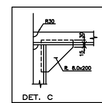
DET. C
