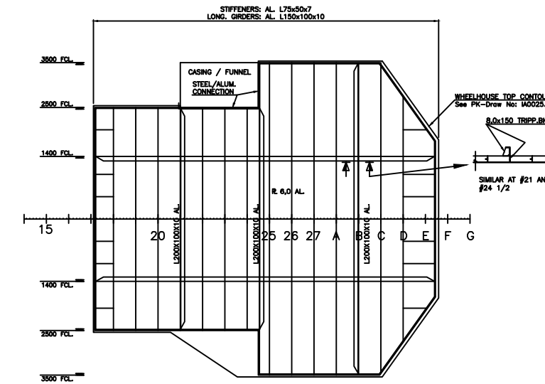
WHEELHOUSE TOP 11400 AB.B.
